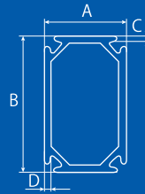
梁:断面図
