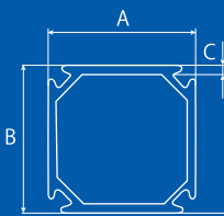
柱:断面図
