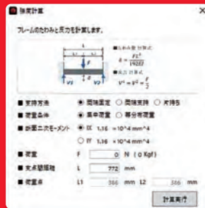
強度計算ウィンドウ
